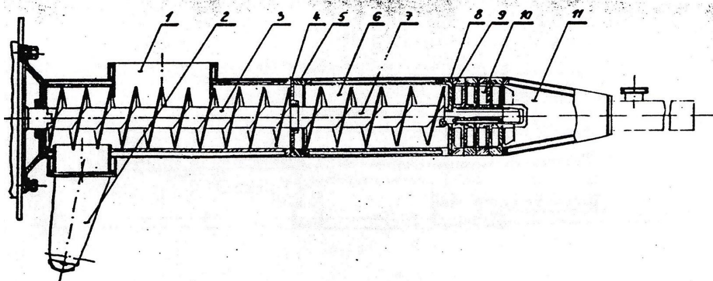
Obr. 52 Schéma miesiča
