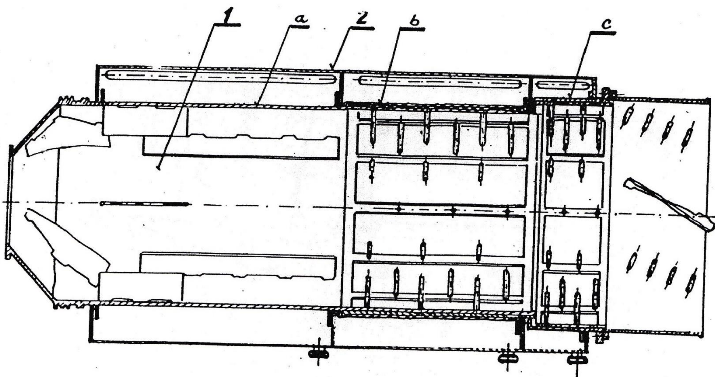
Obr. 51 Schéma odlučovacieho valca
